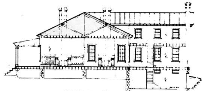
LONGITUDINAL SECTION.
