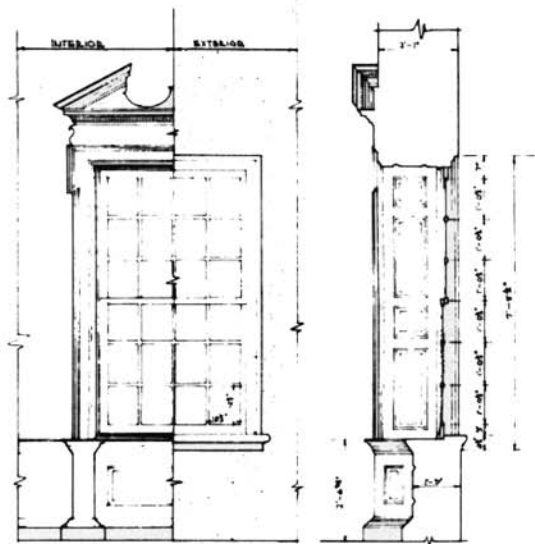
ELEVATION SCALE: 1/2" = 1'-0"
