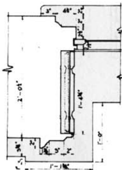
JAMB SCALE: 1/4" = 1'-0"
