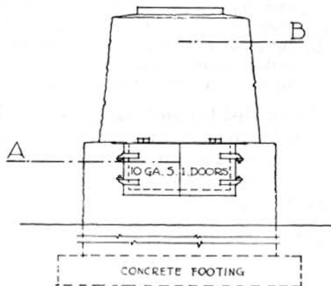
ELEVATION FIG. 3
