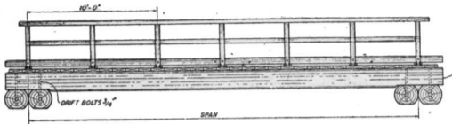
ELEVATION
