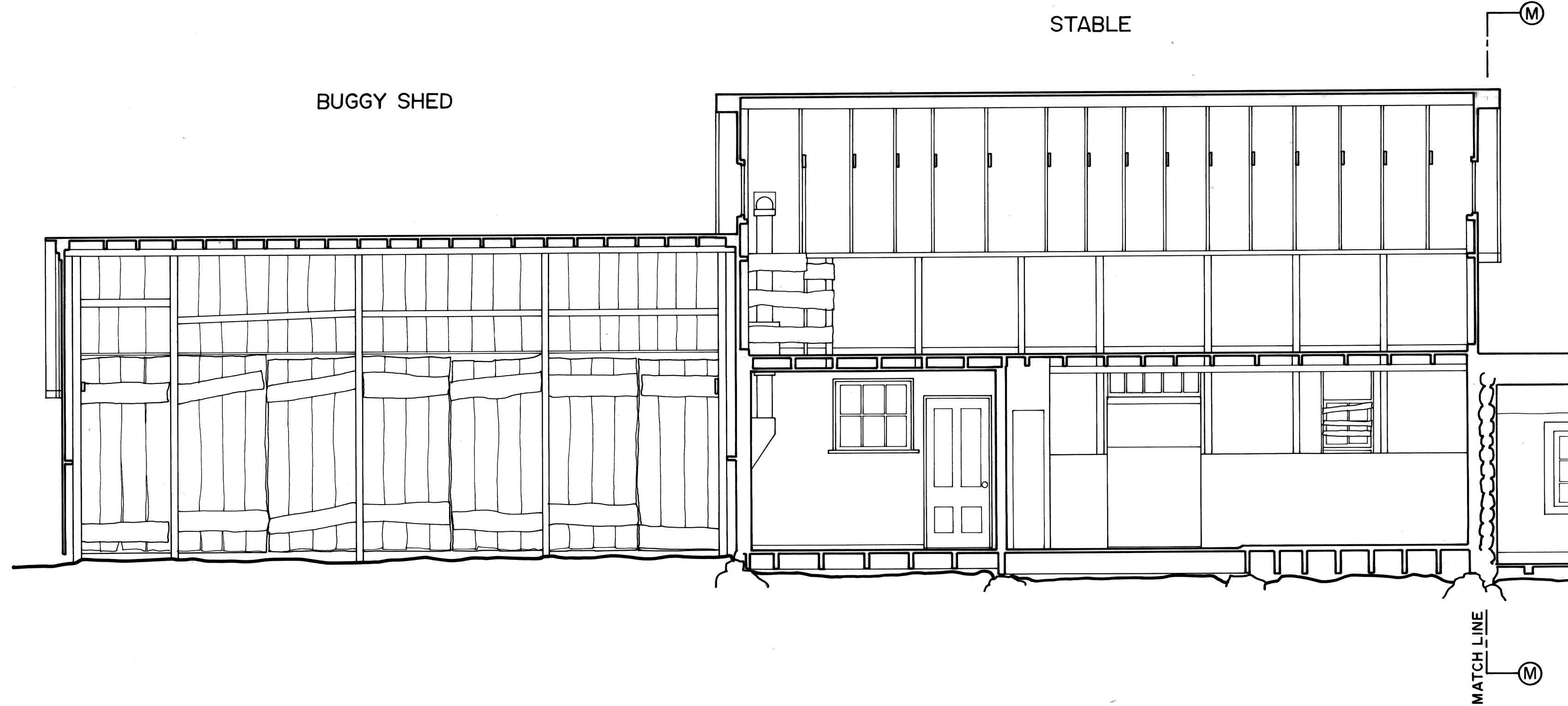
SECTION A-A
