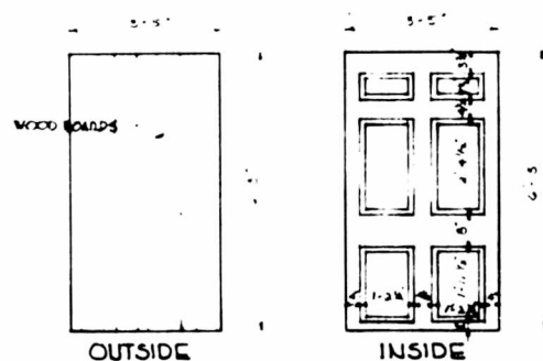
DOOR SCHEDULE
