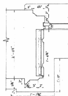
JAMB SCALE: 1/4" = 1'-0"
