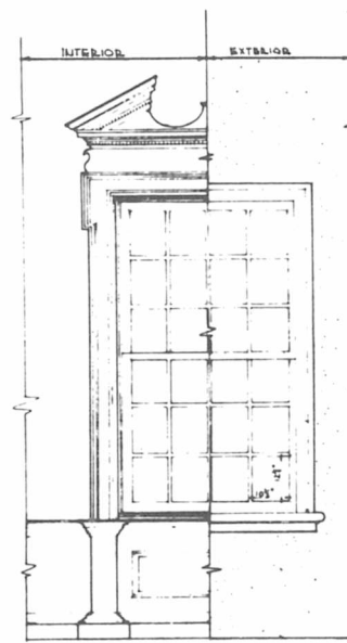
ELEVATION SCALE: 1/2" = 1'-0"
